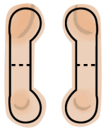
oren
